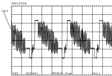
TP 4 : CVBS
