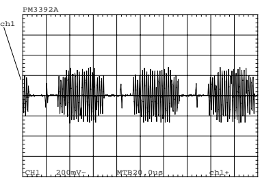
TP 5 : C_ENC
