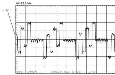
TP 22 : U_VID
