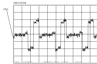
TP 23 : V_VID
